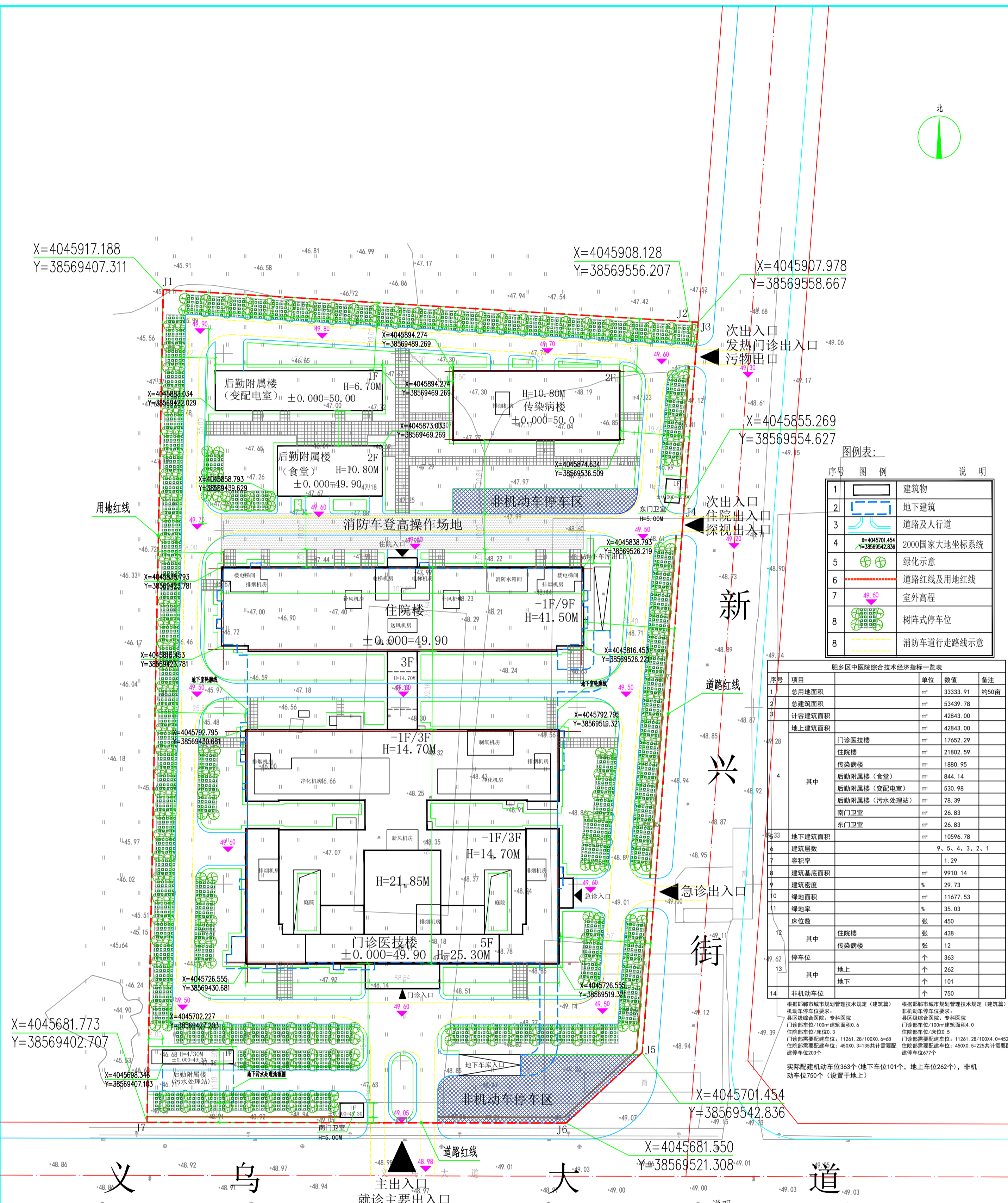
总平面图 1:500
